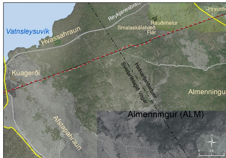
Mynd 6.5 Lega A: Jarðstrengs samhliða Suðurnesjalínu 1 í Almennungi. Rauð punktalína er Suðurnesjalína 2, svört lína er Suðurnesjalína 1 og gular línur eru afmörkun á Almennungi.
