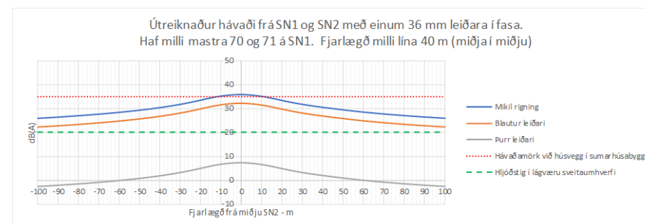
Mynd 20.7 Hávaði frá SN1 og SN2 milli mastra 70 og 71 í SN1, nálægt Vogaaflleggjara. SN2 lögð sem loftlína með einum 36 mm leiðara í fasa (Jón Bergmundsson, 2018).
