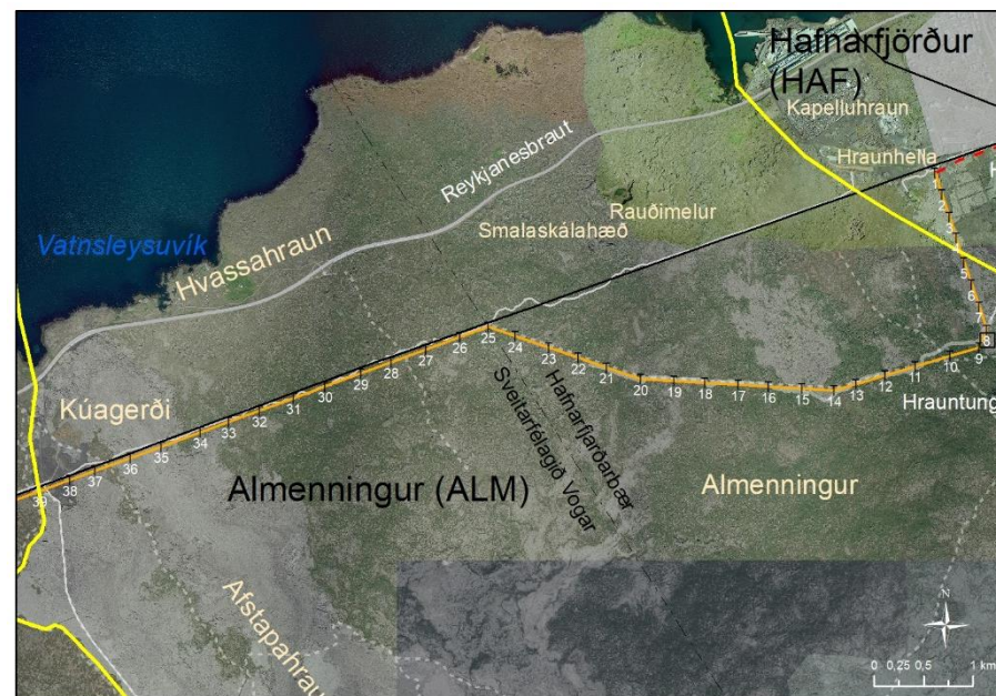
Mynd 6.21 Lega loftlínu í Almenningi.
