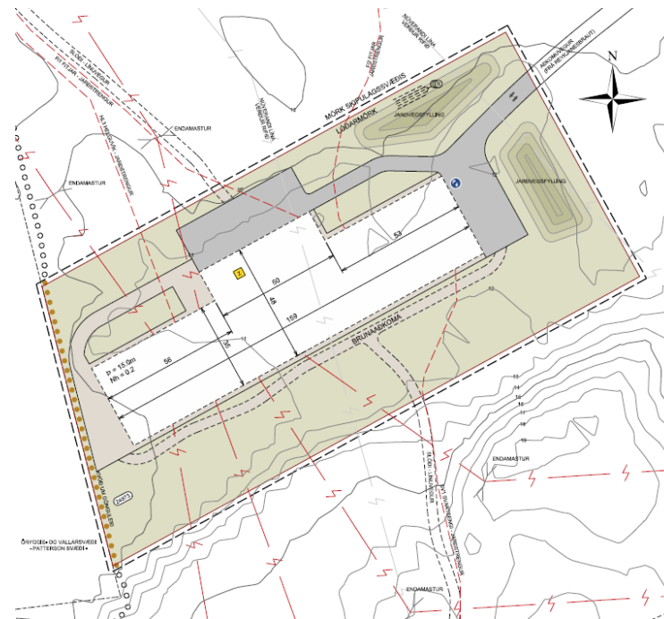
Mynd 5.10 Tengivirki og lóð á Njarðvíkurheiði skv. deiliskipulagi
