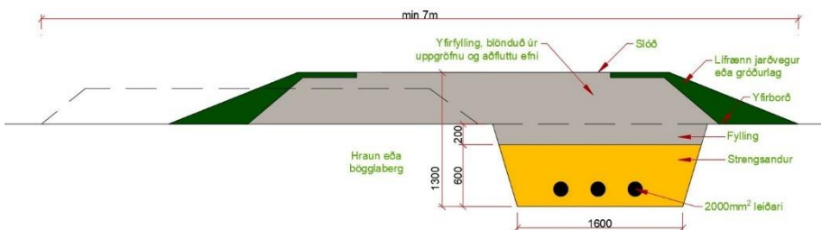
Mynd 5.7 Snið í lítið eða óhreyfðu hrauni (Snið II)
