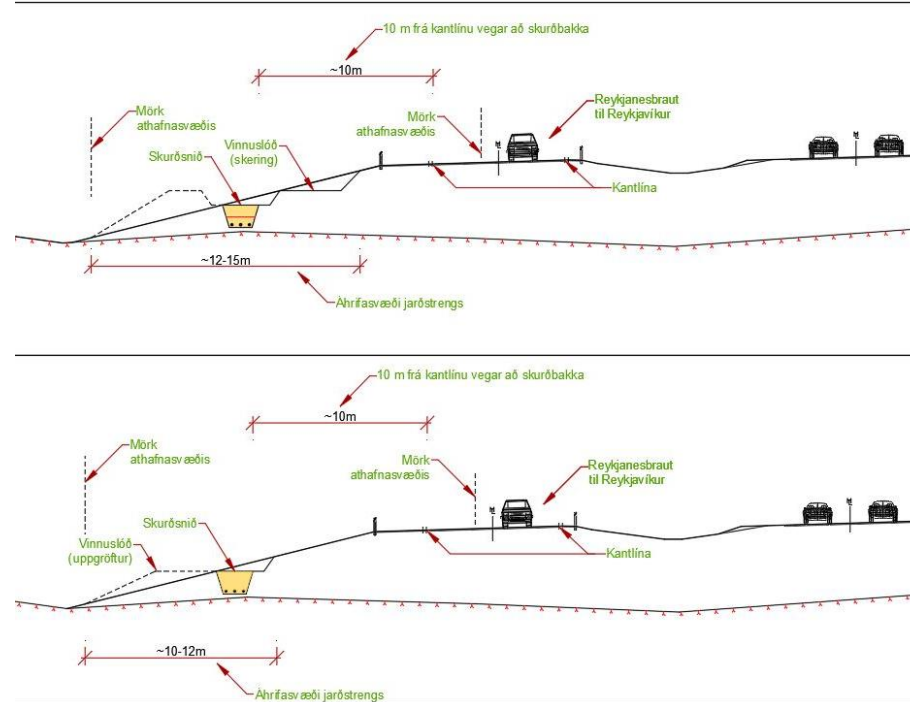
Mynd 6.11 Snið 1 hefðbundið snið og afstaða gagnvart vegi á lágrí fyllingu
