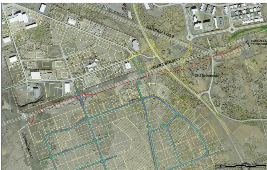
Mynd 6.18 Útfærsla á línu í Hafnarfirði. Lega jarðstrengs ermilli Hamraness og Hraunhelli (rautt brotastrík). Við tekur loftlína með stefnu á Hrauntungur (hvít lína).
