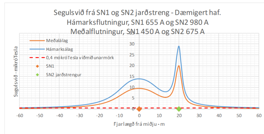
Mynd 20.9 Segulsvið frá SN1 og SN2 jarðstreng, dæmigert haf (Jón Bergmundsson, 2018).
