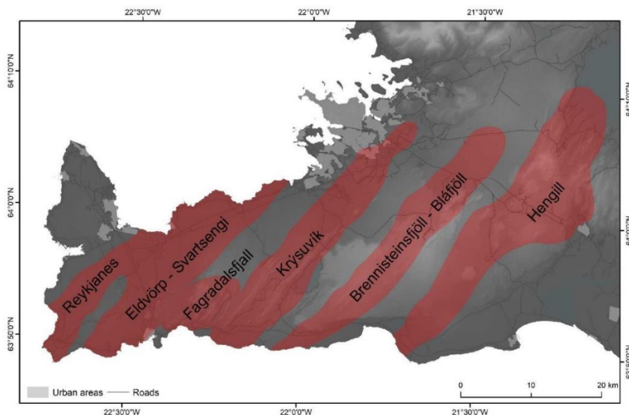
Mynd 21.1 Eldstöðvakerfin á Reykjanesskaga (Ármann Höskuldsson et al, 2018)
