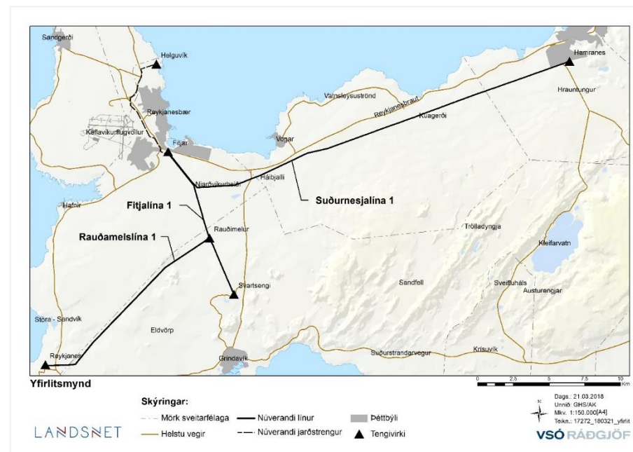
Mynd 2.2 Yfirlitsmynd af núverandi flutningskerfi á Suðurnesjum
