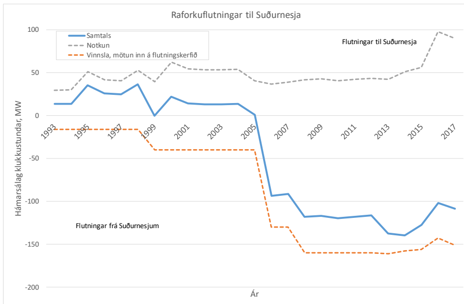
Mynd 2.1 Hámarks klukkutímaág raforkuflutninga til og frá Suðurnesjum sem flytja hefur þurft eftir Suðurnesjalínu 1 inn (+) eða út af svæðinu (-)
