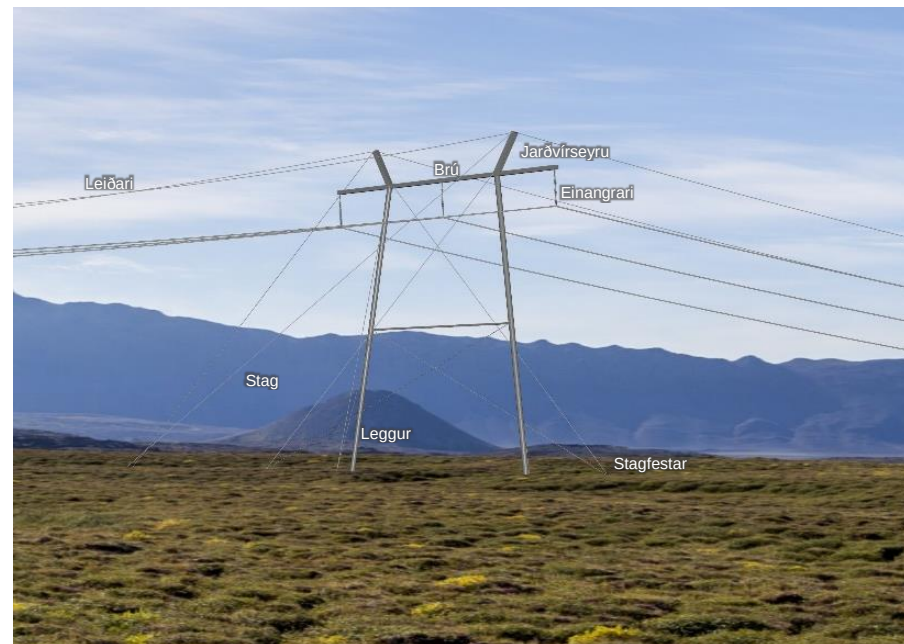
Mynd 5.1 Stagað röramastur með jarðvírseyrum. Helstu hlutar masturs. Efst er brú og millipverslá fyrir miðju sem styður við leggi.
