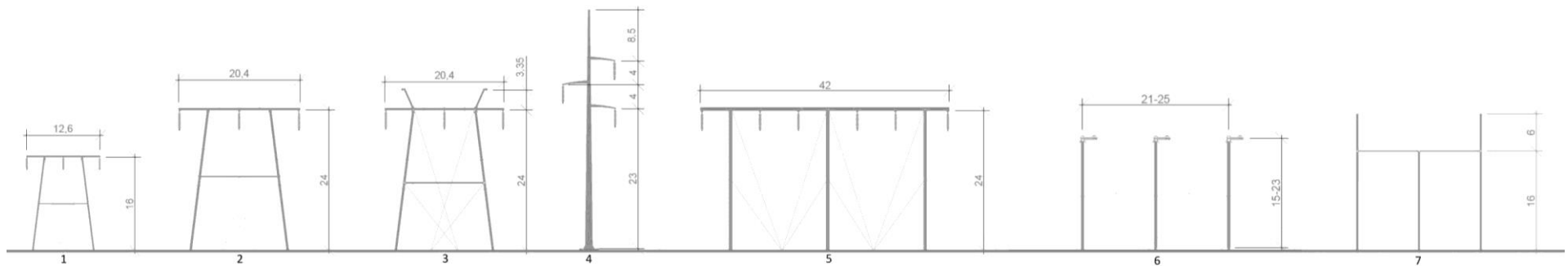
Mynd 5.2 Mastragerðir sem hafa verið til skoðunar í Suðurnesjalínu 2. Sjá einnig Tafla 5.2.
