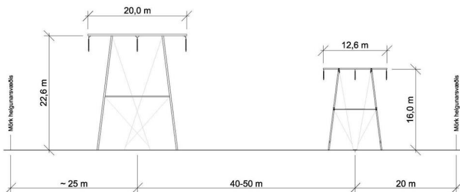
Mynd 5.9 Heildarbreidd helgunarsvæðis þar sem Suðurnesjalína 2 er samsíða Suðurnesjalínu 1 eða Fitjalínu 1
