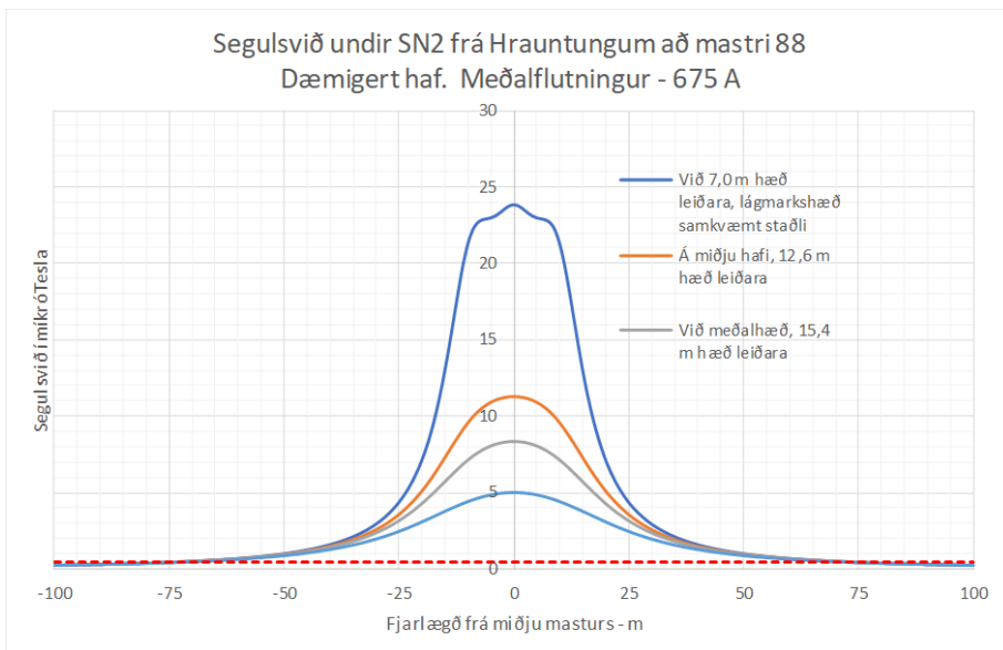
Mynd 20.6 Segulsvið í sniðum þvert á SN2 í dæmigertu hafi við meðalflutning (Jón Bergmundsson, 2018).
