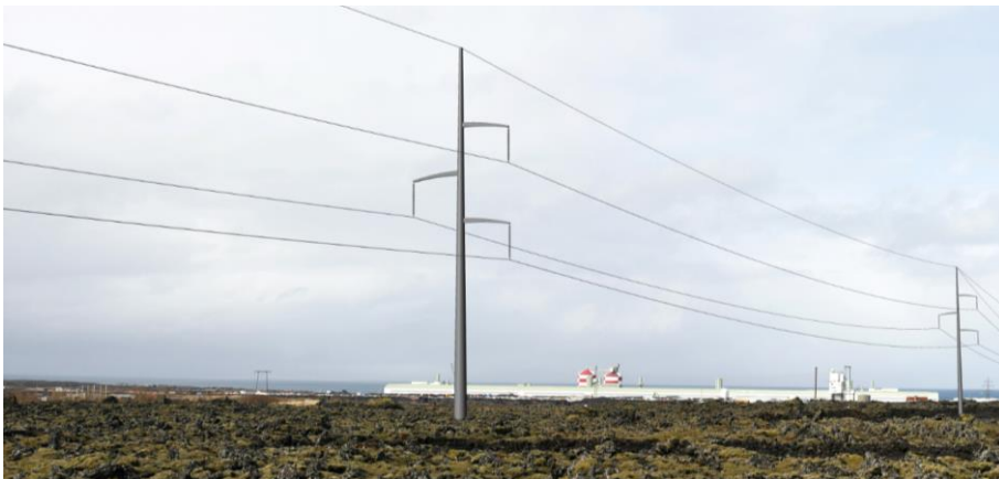
Mynd 6.20 Myndin sýnir útlit súlumastra („þrjóna“) í beltinu frá Hraunhelli að Hrauntungum. Þessi útfærsla krefst mun minna helgunarsvæðis en ef leiðarar eru í láréttri uppröðun.
