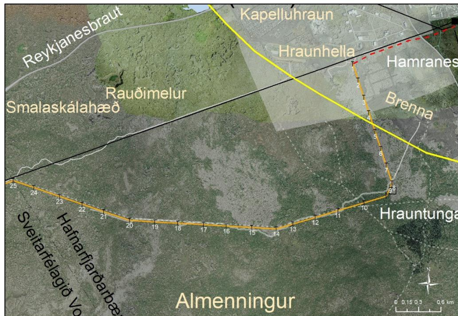
Mynd 6.22 Lega loftlínu í Almningi. Súlumöstur verða frá Hraunhelli að Hrauntungum, möstur nr. 1-8. Jarðstrengur verður frá Hraunhelli að Hamranesi.
