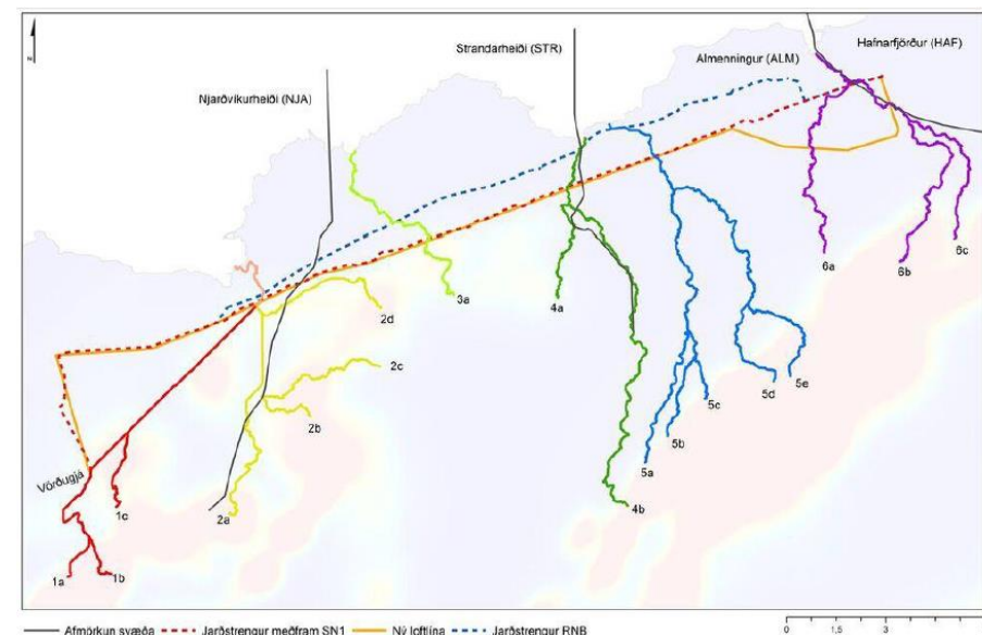
Mynd 21.5 Kort sem sýnir helstu rennislisleiðir hraun er upp koma í eldsumbrotum (Ármann Höskuldsson et al, 2018)
