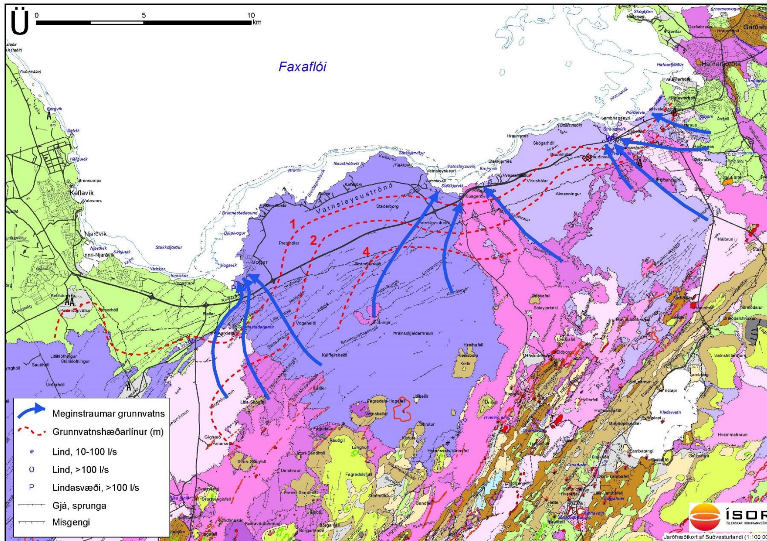
Mynd 16.1 Jarðfræðikort, lindir, grunnvatnshæð og grunnvatnsstraumar. Fjölubláu og bleiku svæðin eru hraun, grænt er grágrýti. (Árni Hjartarson, 2018)
