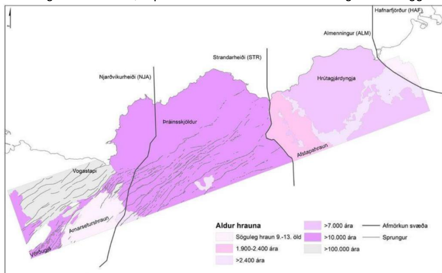
Mynd 21.2 Jarðfræðikort af athugunarsvæðinu. Aldur hrauna og lega gliðnunarprungna og misgengs á fyrirhuguðum línustæðum. (Ármann Höskuldsson et al, 2018)
