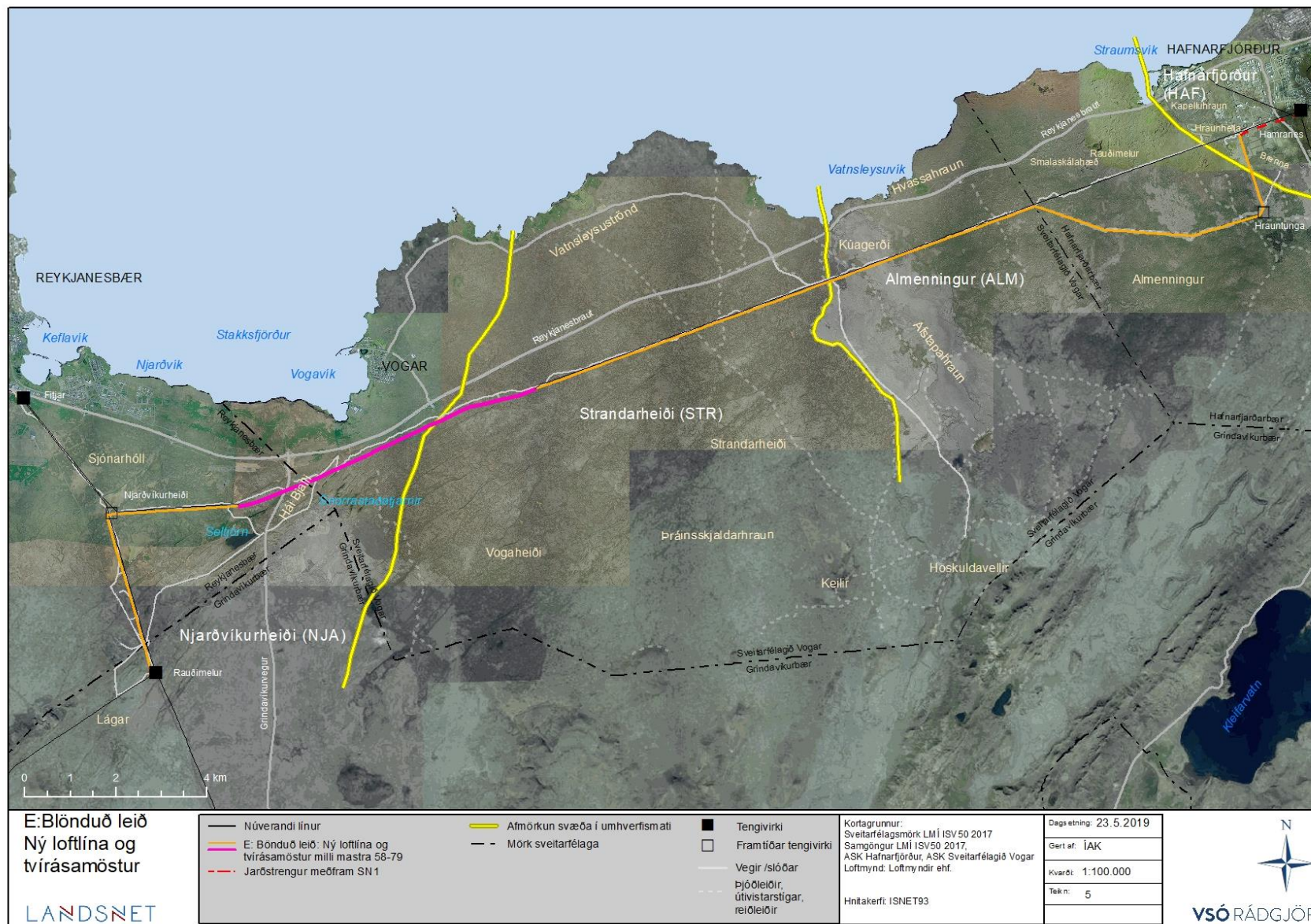
Mynd 6.34 Valkostur E | Blönduð leið loftlínu og tvírásmasturs með Suðurnesjalínu 1 og 2
