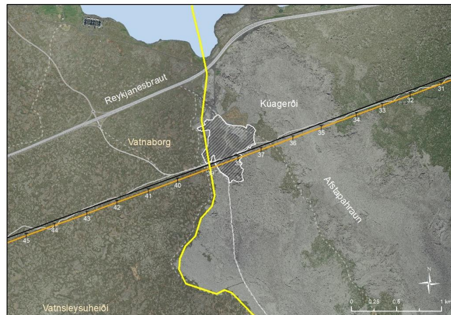
Mynd 6.25 Tillaga að lagersvæði í Afstapahrauni.
